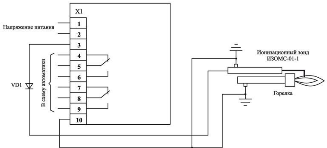
Схема внешних соединений датчиков-реле контроля пламени с использованием эффекта проводимости пламени ДПЗ-71DIN
