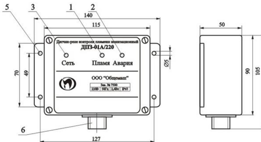
ДПЗ-01А/24, ДПЗ-01А/220
