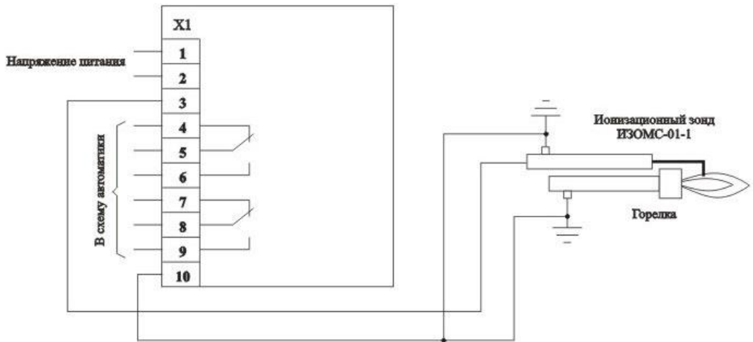
Схема внешних соединений датчиков-реле контроля пламени ДПЗ-01А
