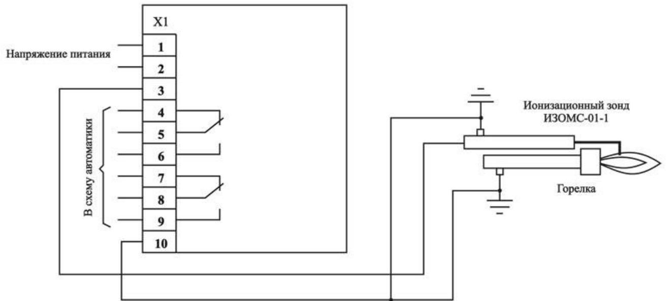
Схема внешних соединений датчиков-реле контроля пламени ДПЗ-71DIN
