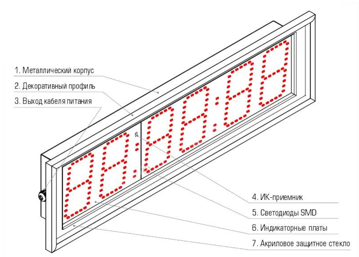
Рис. 1. Типовая конструкция офисных электронных часов Импульс-431-HMS
