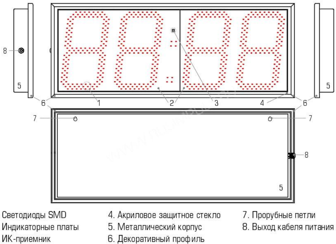
Рис. 2. Типовой чертеж офисных электронных часов «Импульс-410»
