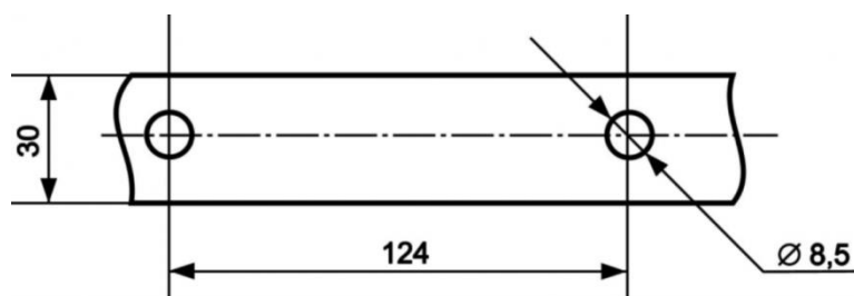
Рис. 2. Размеры отверстий крепления на скобе
