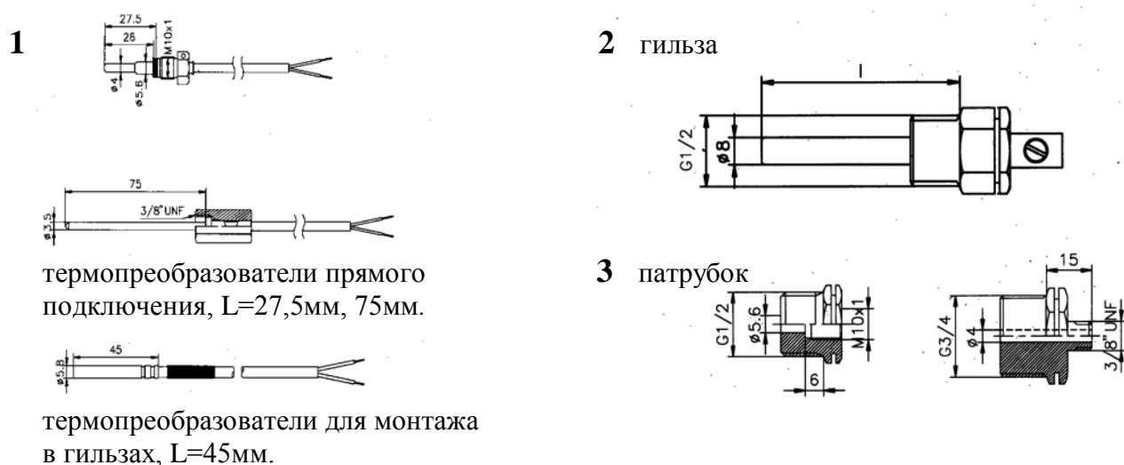
Рис. 2. Термопреобразователи сопротивления.
