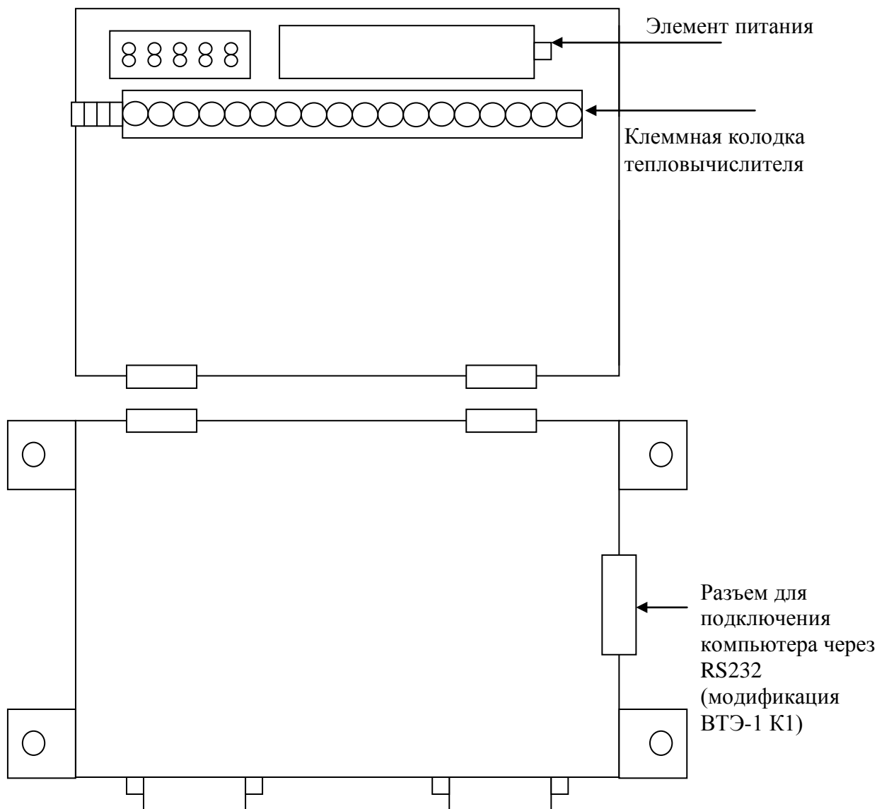
Рис. 5. Вид тепловычислителя с откинутой верхней крышкой.
