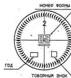
ВИД СНИЗУ
