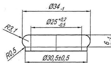
Венчик Масштаб 2:1
