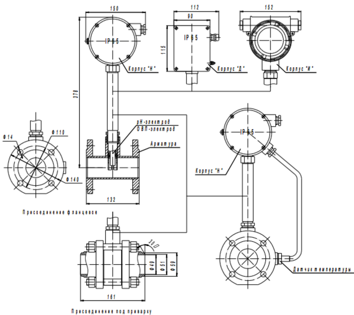
Рис. 1. Арматура магистральная АМН-1.1
