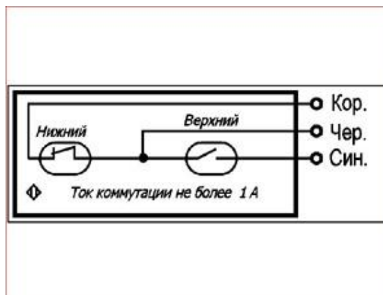
Схема подключения поплавкового датчика уровня ВБУ-32
