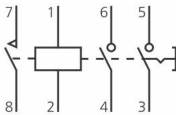
б) РЭУ11-30
