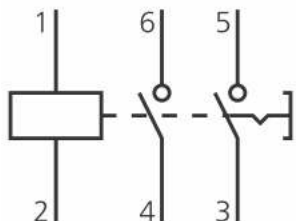
а) РЭУ11-20
