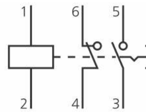
в) РЭУ11-11
