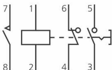
г) РЭУ11-21
