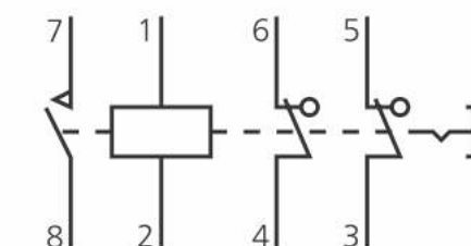
е) РЭУ11-12
