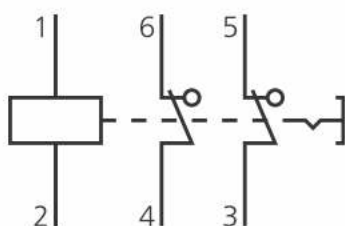
д) РЭУ11-02
