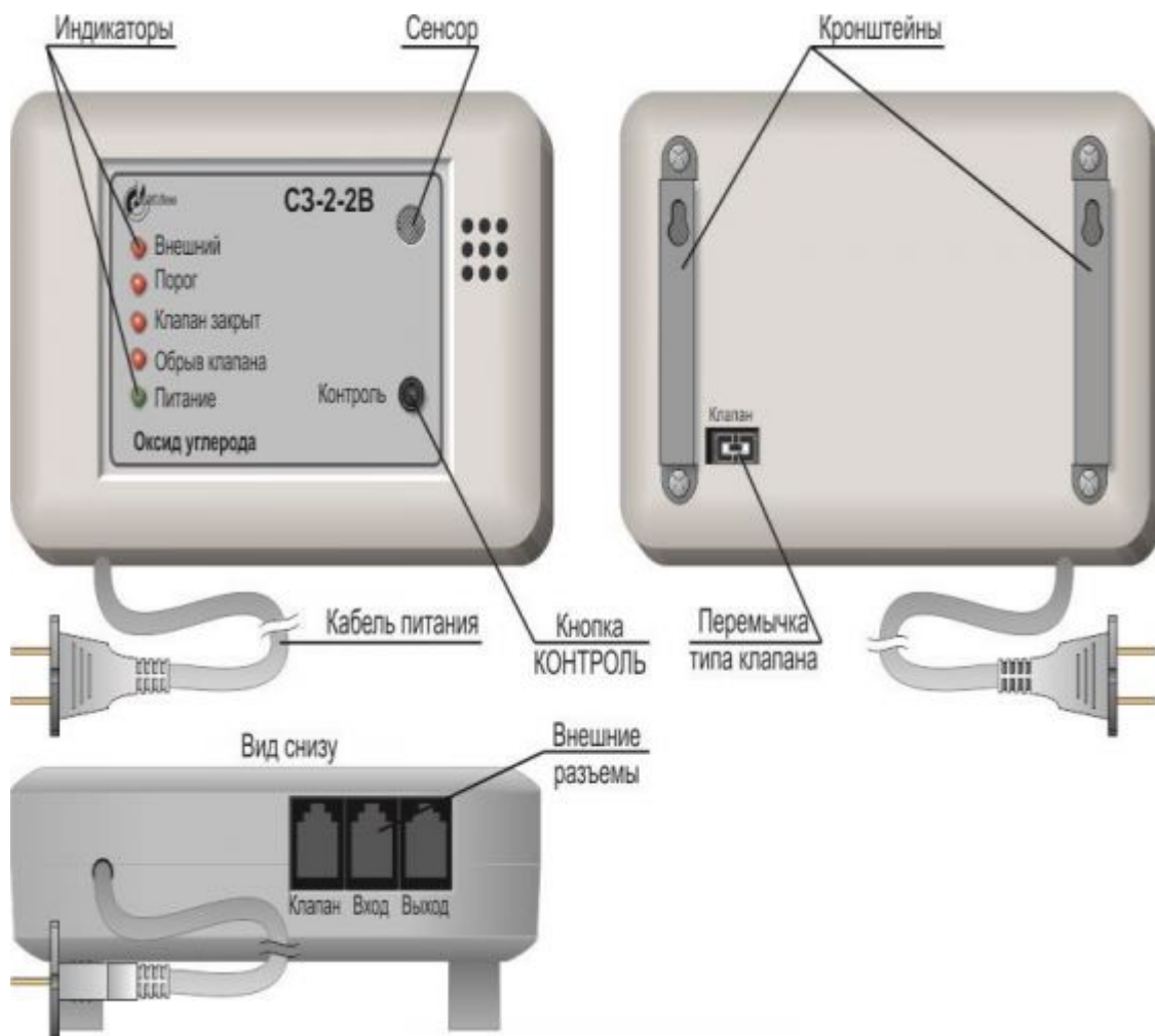
Рис1. Сигнализатор С3-2-2В
