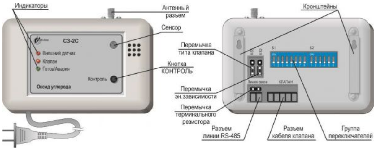
Рис3. Сигнализатор СЗ-2С
