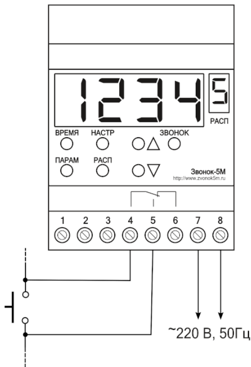
Подключение к существующей кнопке подачи звонков
