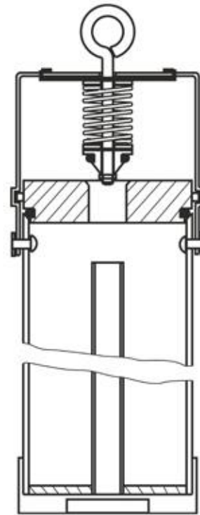
ПО-2У
