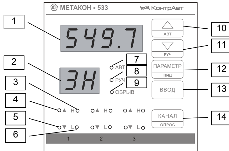
Рисунок 22 – Лицевая панель приборов серии «Метакон-533»
