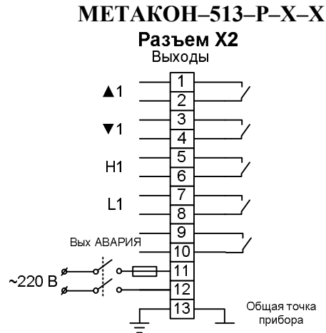
Рисунок 11 – Схемы подключения выходных цепей к клеммным соединителям для модификаций МЕТАКОН-513-Р-Х-Х
