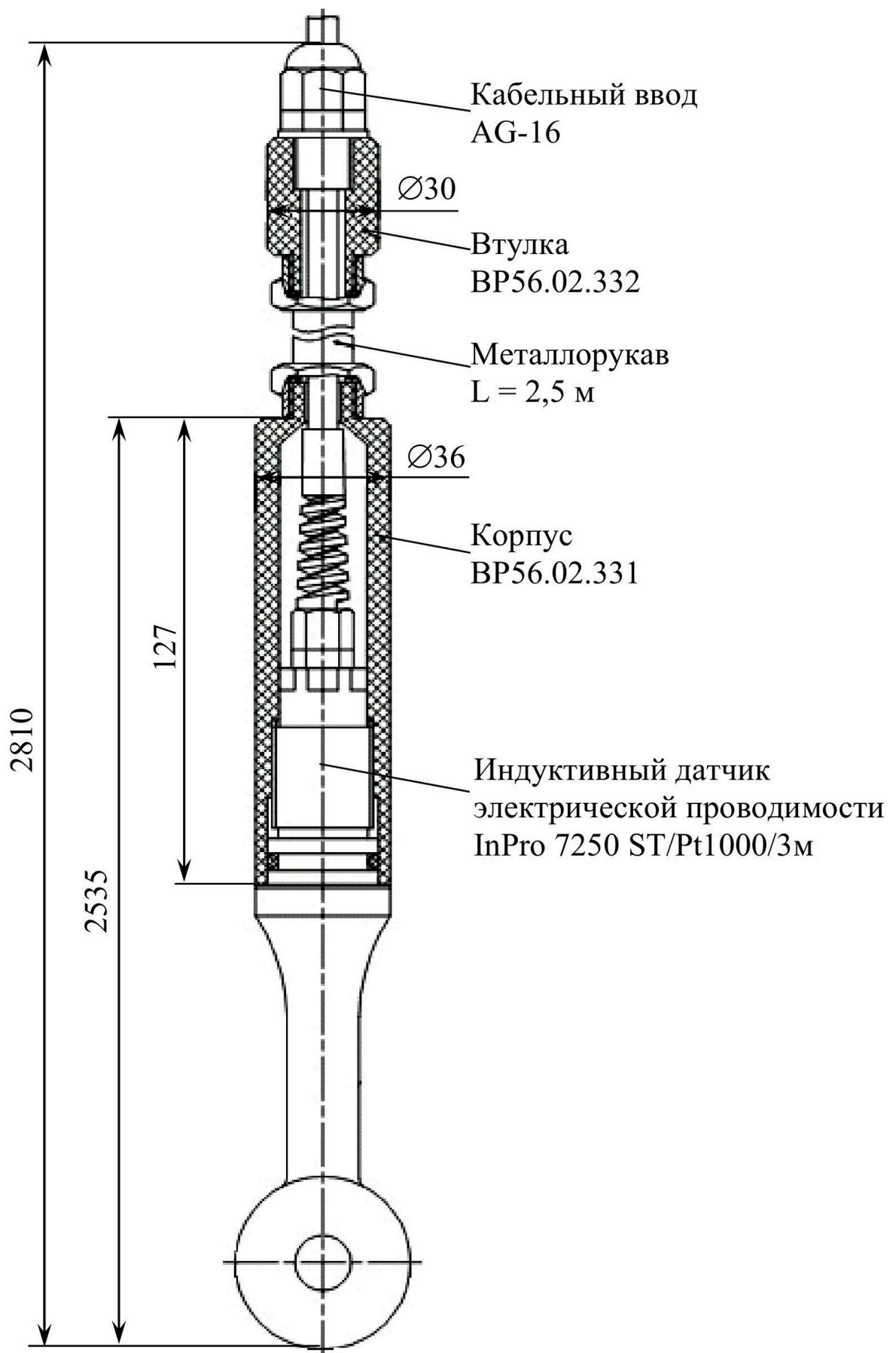
Датчик проводимости для проведения измерений на глубине
