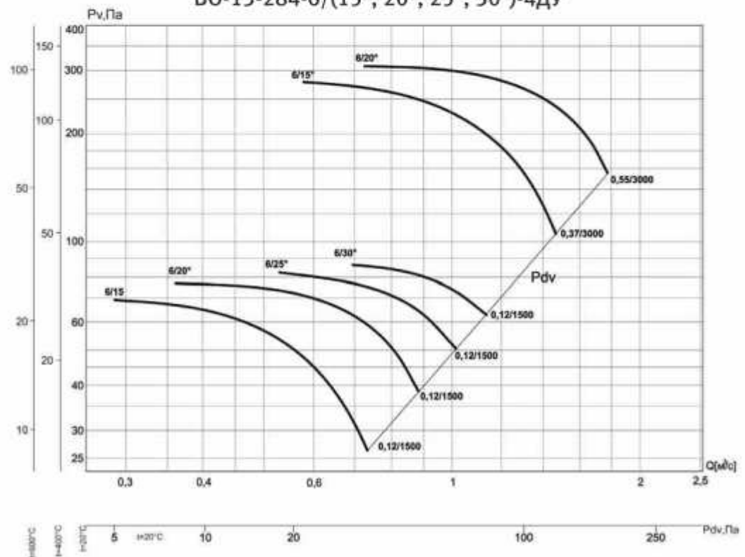
ВО-13-284-6/(15°, 20°, 25°, 30°)-4ДУ
