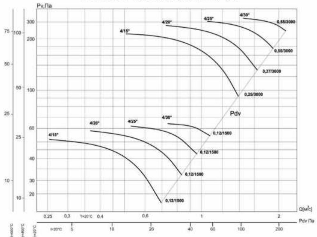
ВО-13-284-6/(15°, 20°, 25°, 30°)-4ДУ
