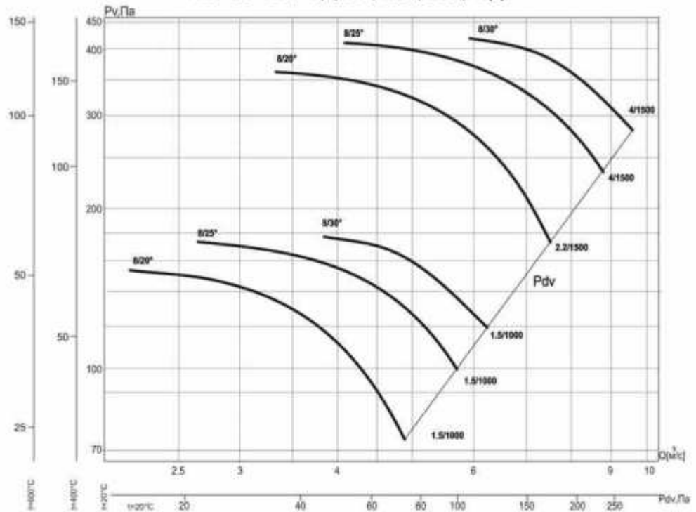
ВО-13-284-8/(20°, 25°, 30°)-8ДУ
