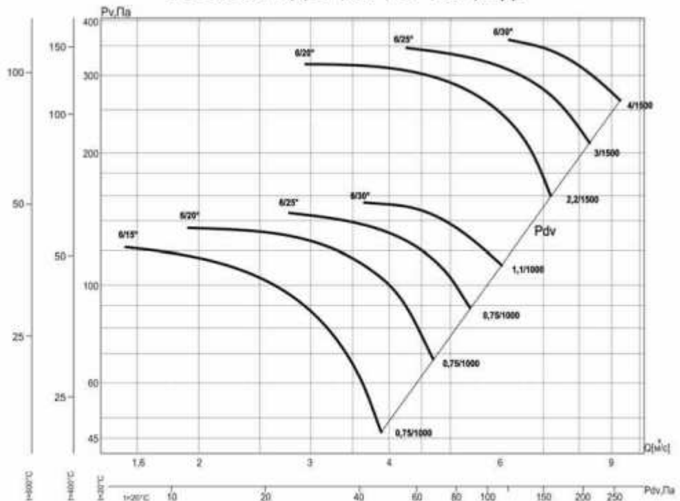
ВО-13-284-6/(15°, 20°, 25°, 30°)-8ДУ
