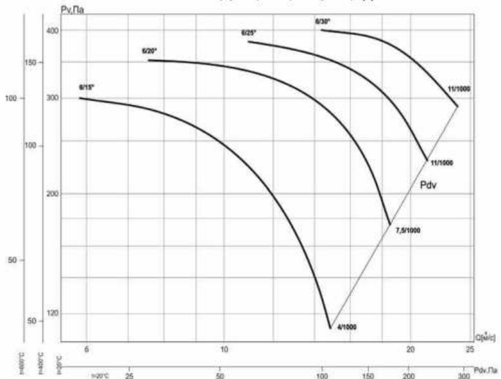
ВО-13-284-6/(20°, 25°, 30°)-12,5ДУ
