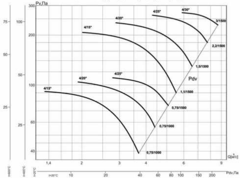
ВО-13-284-4/(15°, 20°, 25°, 30°)-8ДУ
