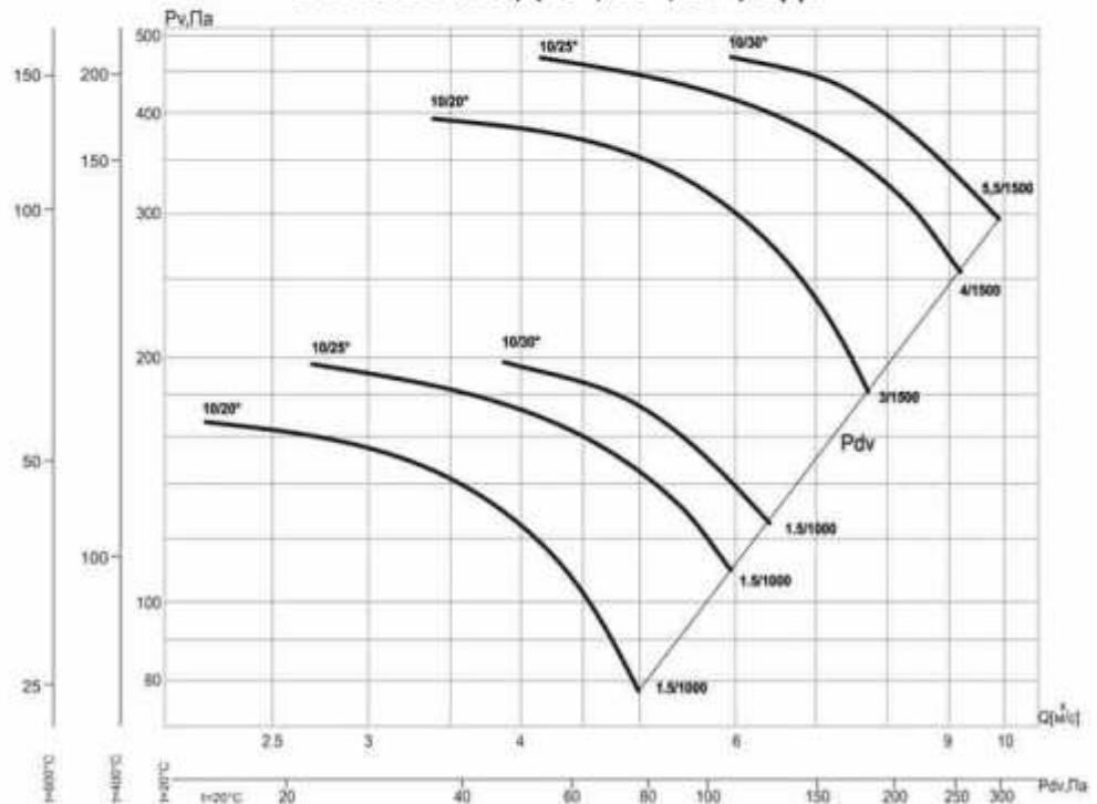
ВО-13-284-10/(20°, 25°, 30°)-8ДУ
