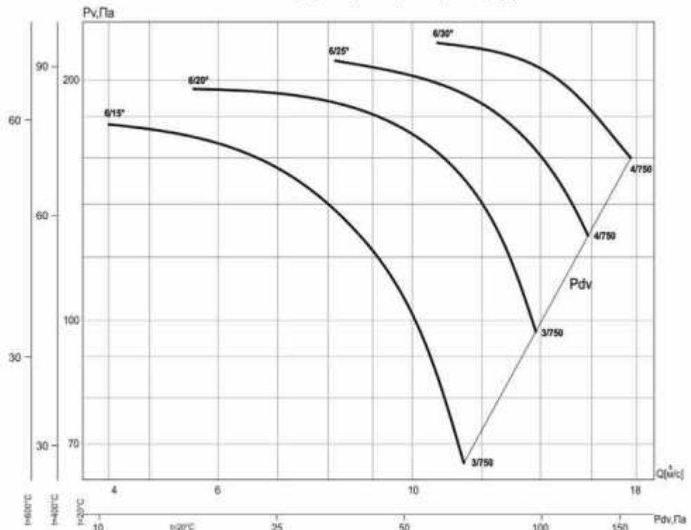
ВО-13-284-6/(20°, 25°, 30°)-12,5ДУ
