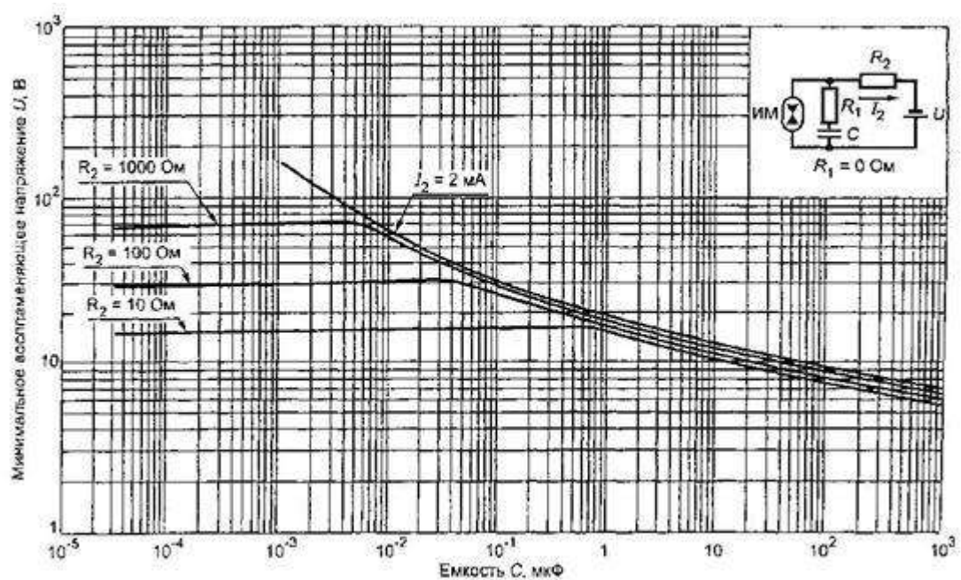
Рисунок А.16. Минимальное воспламеняющее напряжение в активизированной взрывоопасной водородно-кислородной смеси (75 % H_2 + 25 % O_2 ) для емкостных цепей подгруппы IIB при R_1 = 0 \text{ Ohm}
