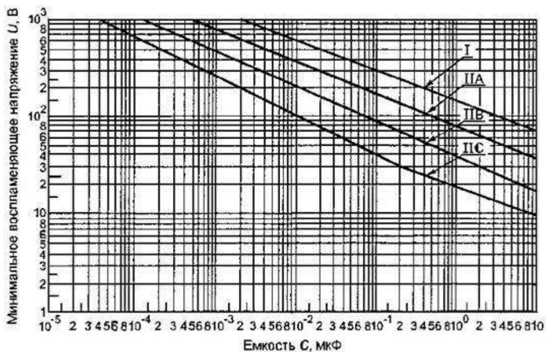
Рисунок А1.6. Емкостные цепи для группы I и подгрупп IIA, IIB, IIC
