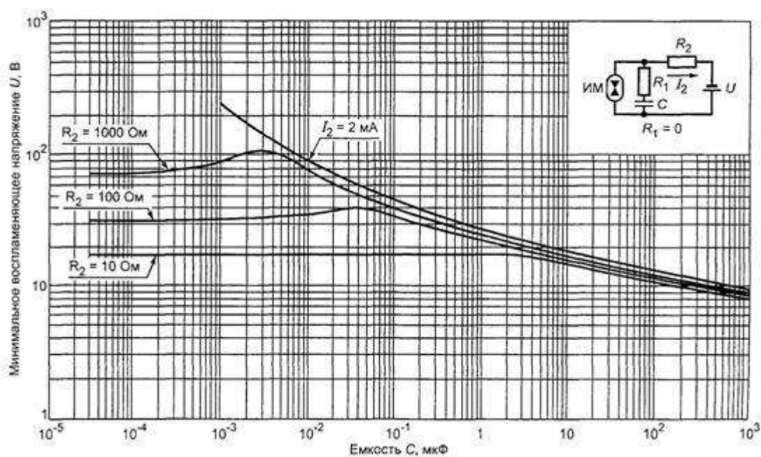
Рисунок А.12. Минимальное воспламеняющее напряжение в активизированной взрывоопасной водородно-кислородной смеси (81 % H_2 + 19 % O_2 ) для емкостных цепей подгруппы IIA при R_1 = 0 \Omega
