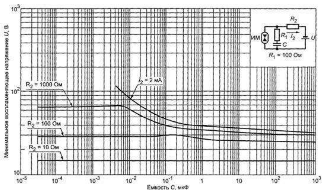
Рисунок А.18. Минимальное воспламеняющее напряжение в активизированной взрывоопасной водородно-кислородной смеси (75 % H_2 + 25 % O_2 ) для емкостных цепей подгруппы IIB при R_1 = 100 \text{ Ом}
