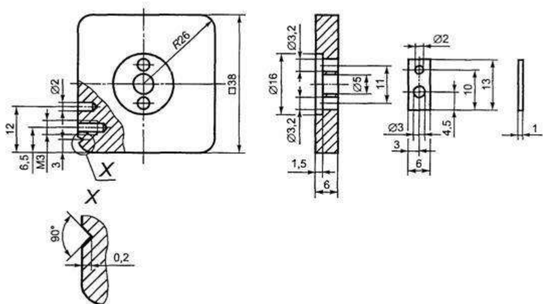
Рисунок Б.3. Держатель проволочек
