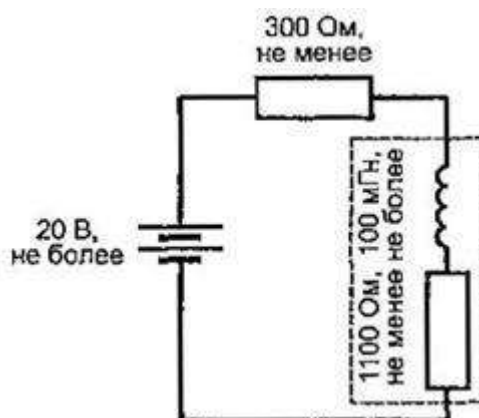
Рисунок А.23. Простая индуктивная цепь
