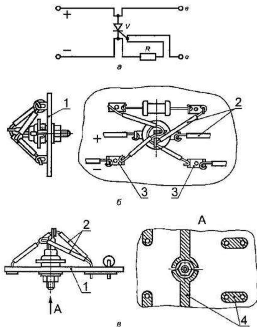
а - электрическая схема; б - навесной монтаж; в - печатный монтаж; V - шунтирующий тиристор; R - токоограничительный резистор, е - к искробезопасной цепи (шунтирующему элементу); 1 - панель; 2 - провод; 3 - лепесток; 4 - печатный проводник
