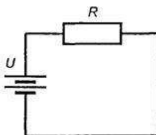
Рисунок А.25. Простая омическая цепь
