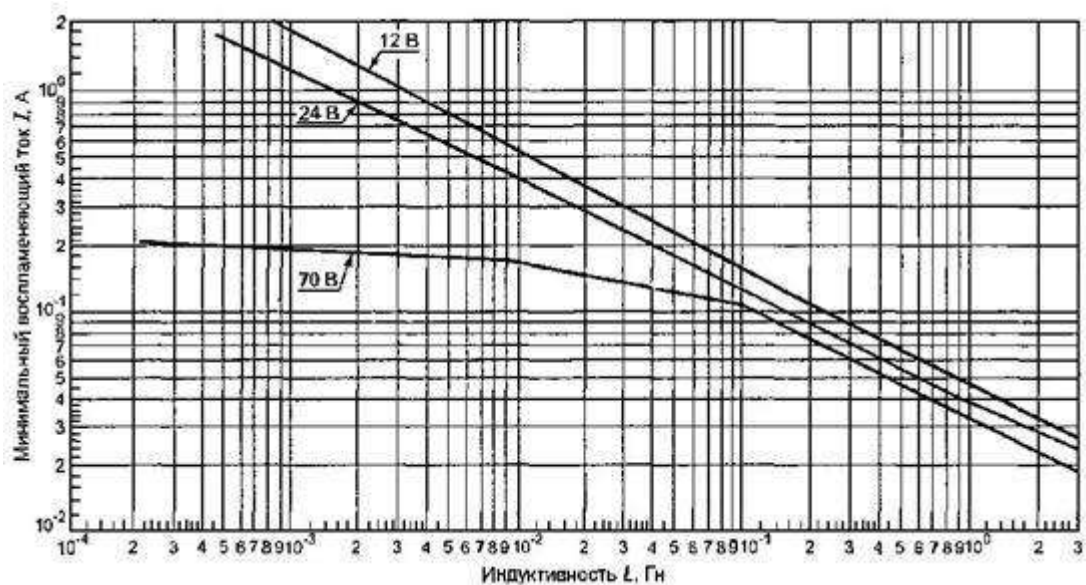
Рисунок А.6. Индуктивные цепи подгруппы ИС
