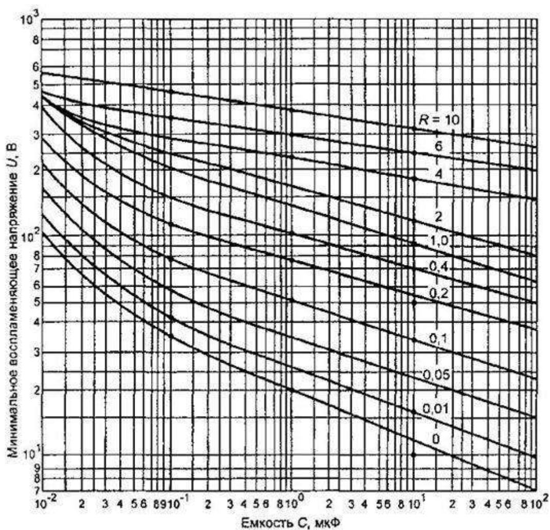
Рисунок А1.9. Зависимость минимального воспламеняющего напряжения от емкости цепи и сопротивления ограничительного резистора для этиленовоздушной смеси
