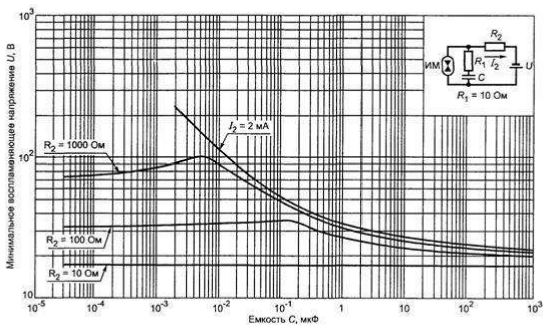
Рисунок А.13. Минимальное воспламеняющее напряжение в активизированной взрывоопасной водородно-кислородной смеси (81 % H_2 + 19 % O_2 ) для емкостных цепей подгруппы IIA при R_1 = 10 \Omega
