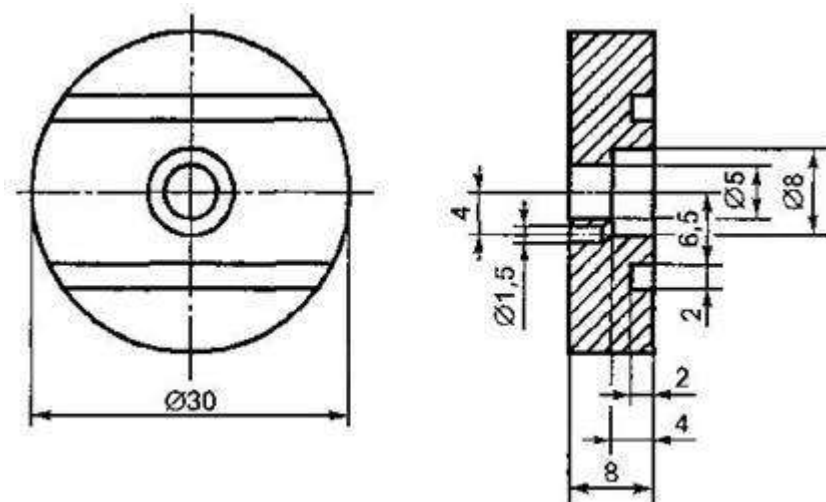
Рисунок Б.2. Кадмиевый контактный диск
