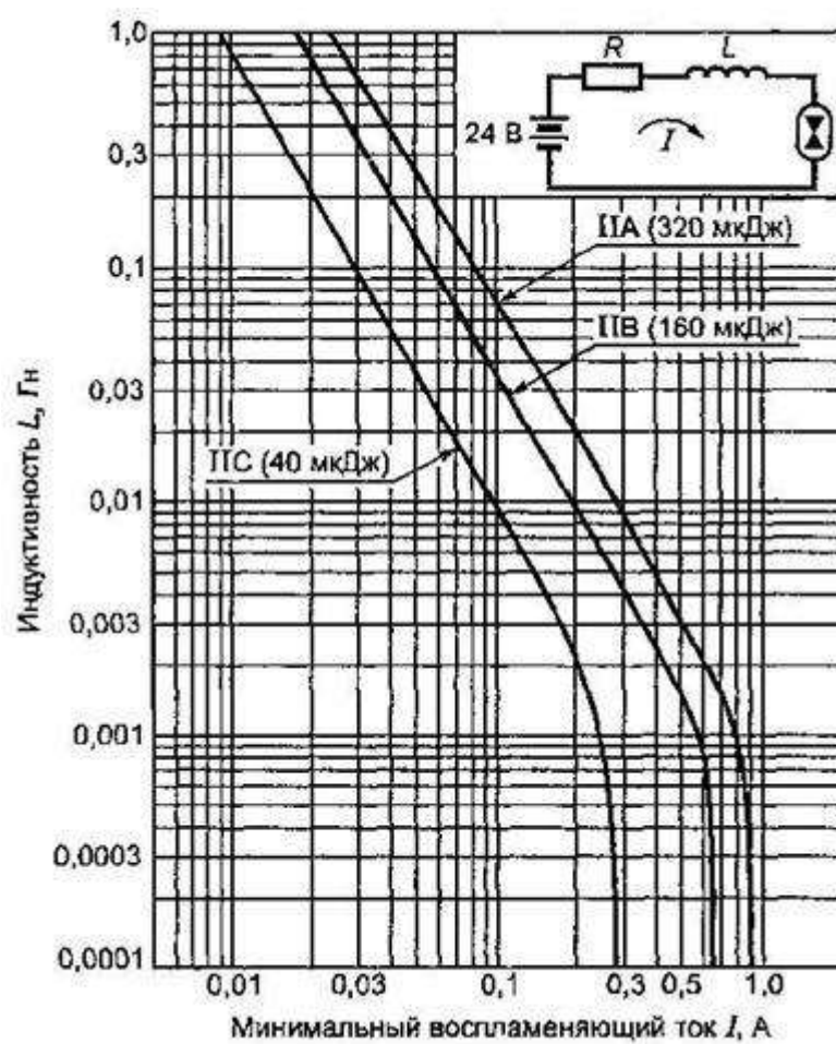
Рисунок А.3. Емкостные цепи группы II
