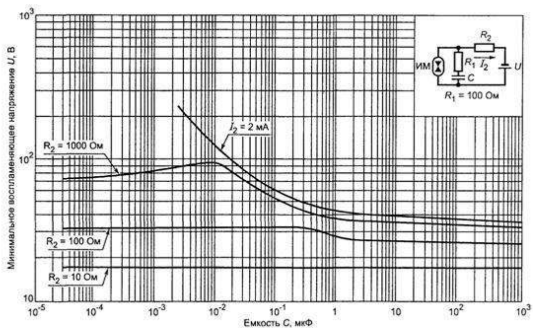
Рисунок А.14. Минимальное воспламеняющее напряжение в активизированной взрывоопасной водородно-кислородной смеси (81 % \text{H}_2 + 19 % \text{O}_2 ) для емкостных цепей подгруппы IIA при R_1 = 100\ \Omega
