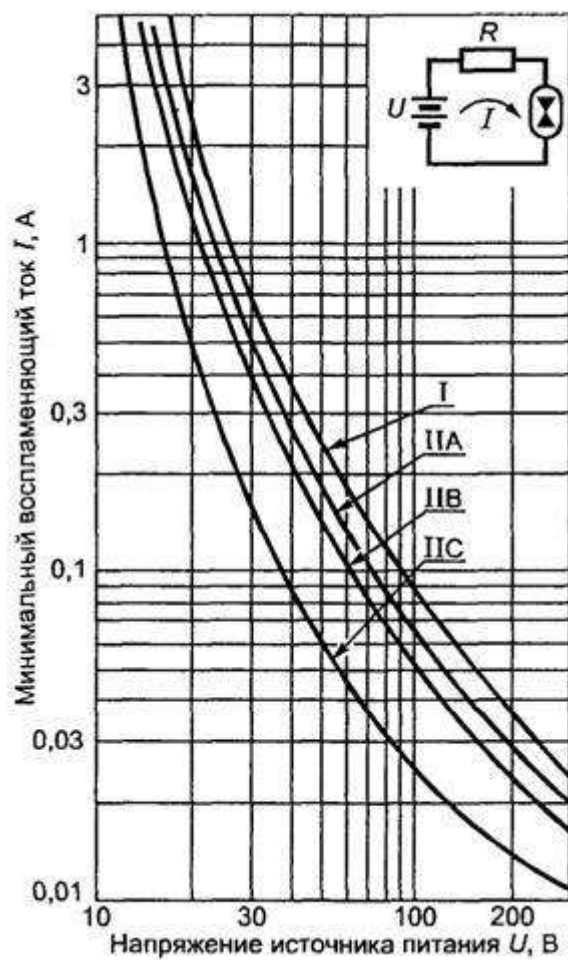
Рисунок А.1. Омические цепи
