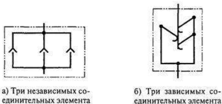
Рисунок 2. Примеры автономных и неавтономных соединительных элементов
