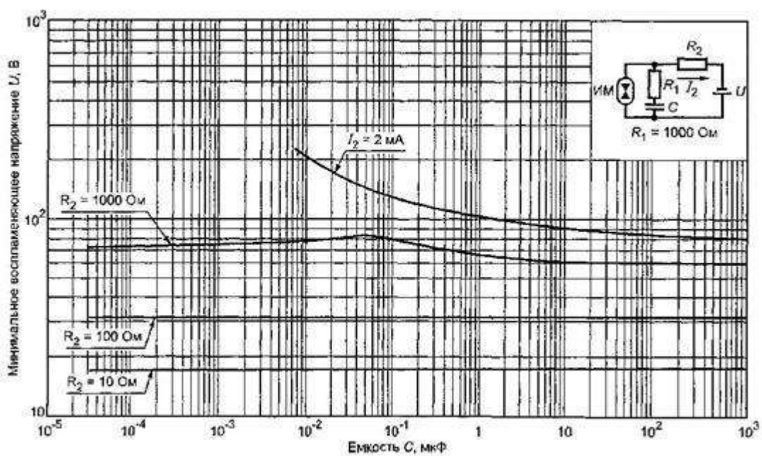
Рисунок А.15. Минимальное воспламеняющее напряжение в активизированной взрывоопасной водородно-кислородной смеси (81 % \text{H}_2 + 19 % \text{O}_2 ) для емкостных цепей подгруппы IIA при R_1 = 1000\ \Omega
