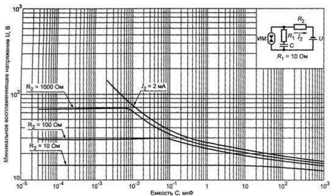
Рисунок А.17. Минимальное воспламеняющее напряжение в активизированной взрывоопасной водородно-кислородной смеси (75 % H_2 + 25 % O_2 ) для емкостных цепей подгруппы IIB при R_1 = 10 \text{ Ohm}
