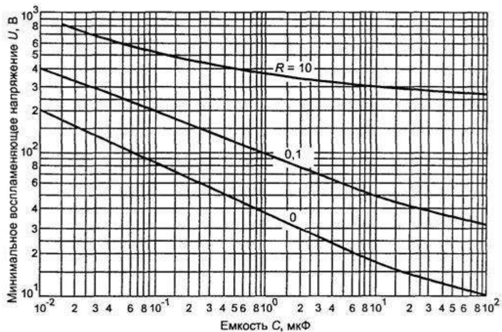
Рисунок A1.8. Зависимость минимального воспламеняющего напряжения от емкости цепи и сопротивления ограничительного резистора для пентановоздушной смеси
