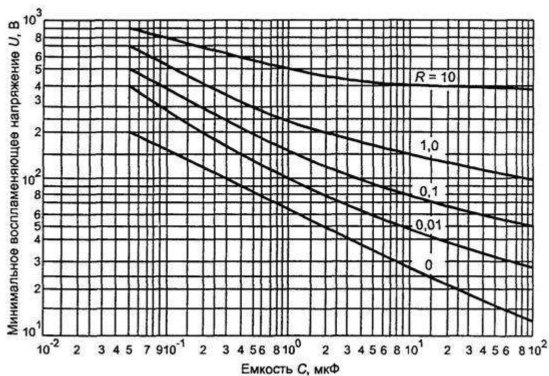
Рисунок A1.7 Зависимость минимального воспламеняющего напряжения от емкости цепи
