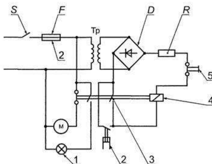
Рисунок Б.5. Пример датчика давления взрыва
