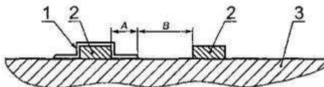
1 - лак; 2 - проводник; 3 - подложка
