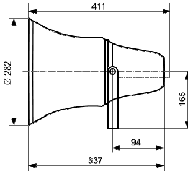
Габаритные размеры
