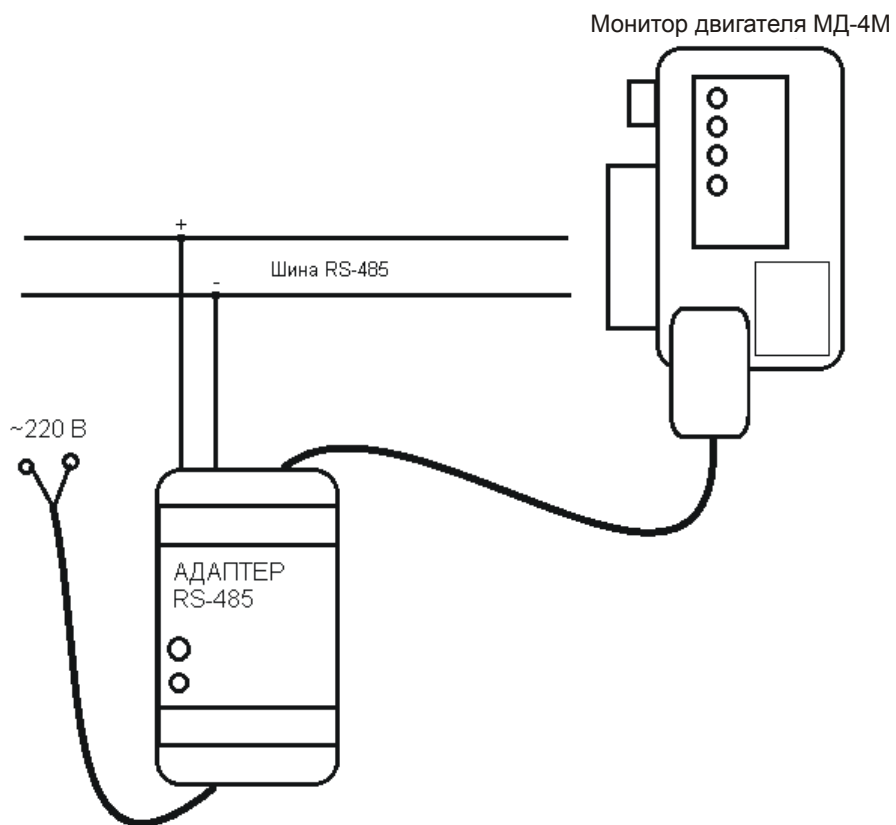
Рисунок 26 – подключение адаптера RS-232
