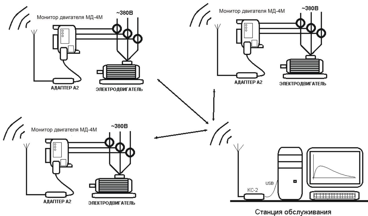
Рисунок 28 – схема организации связи в сети беспроводного доступа
