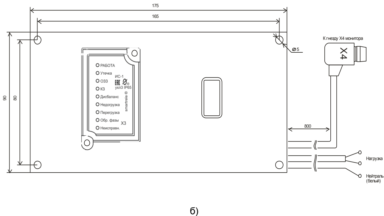
Рисунок 19 – модуль ИС1 а) без панели, б) с панелью
