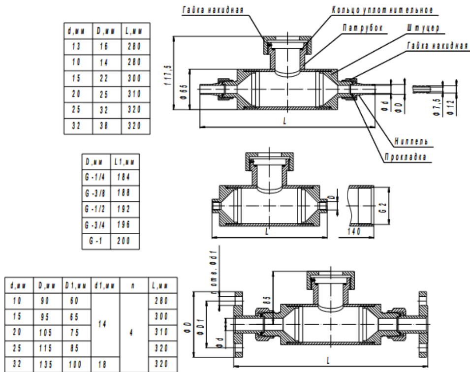
Рис. 2. Арматуры магистральные АМП-1.3
