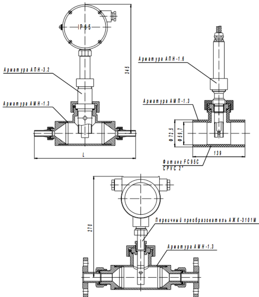
Рис. 3. Примеры использования арматур магистральных АМН-1.3; АМП-1.3
