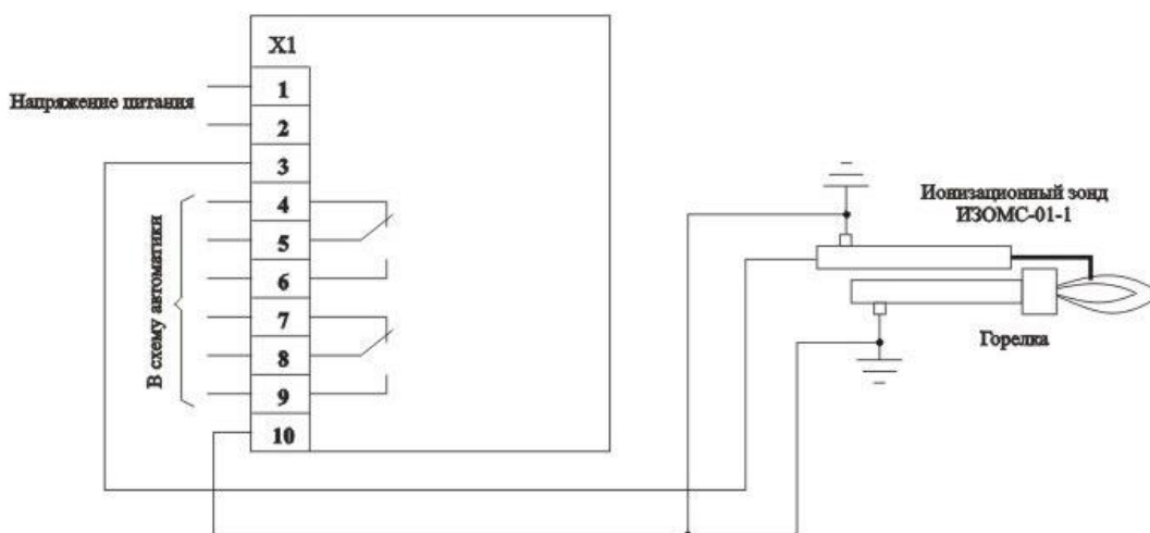
Схема внешних соединений датчиков-реле контроля пламени ДПЗ-01А
