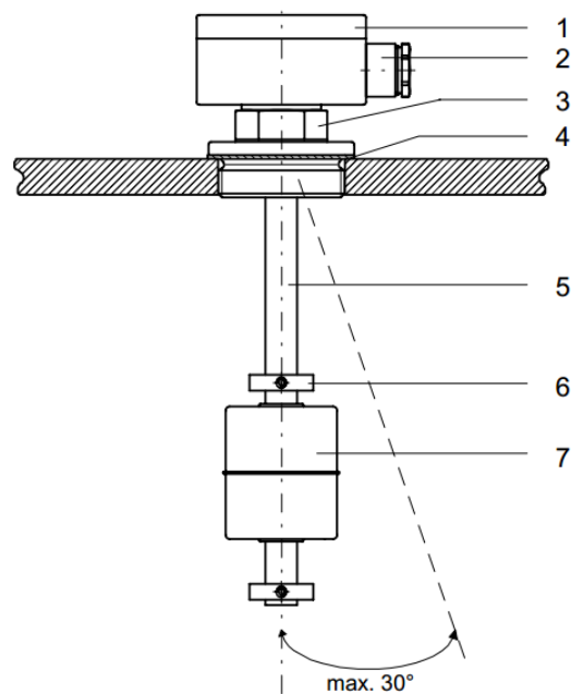
Рисунок 1.2 Монтаж сигнализатора вертикального исполнения
