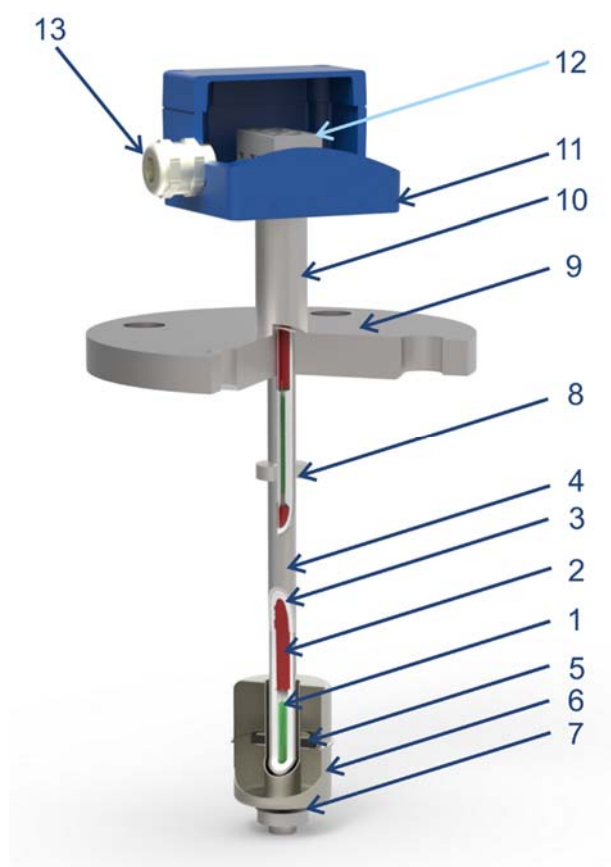
Рисунок 1.1 Устройство сигнализатора уровня LLS-F-T
