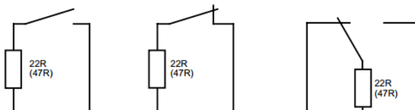
Рисунок 1.4 Подключение защитных сопротивлений
