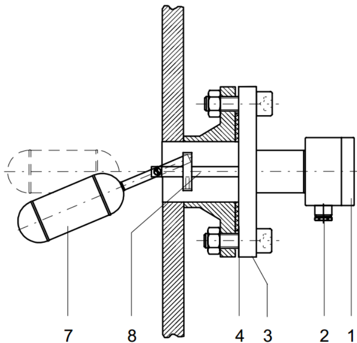
Рисунок 3.2 Монтаж сигнализатора горизонтального исполнения.
