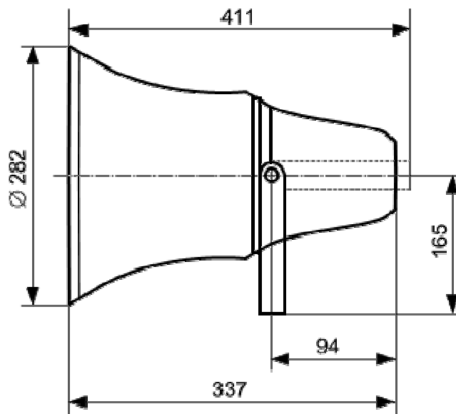
Габаритные размеры
